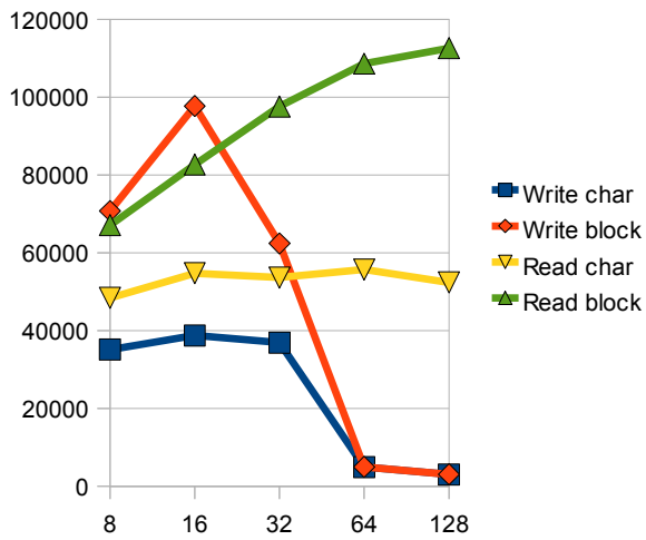
RAID5 3HDD
